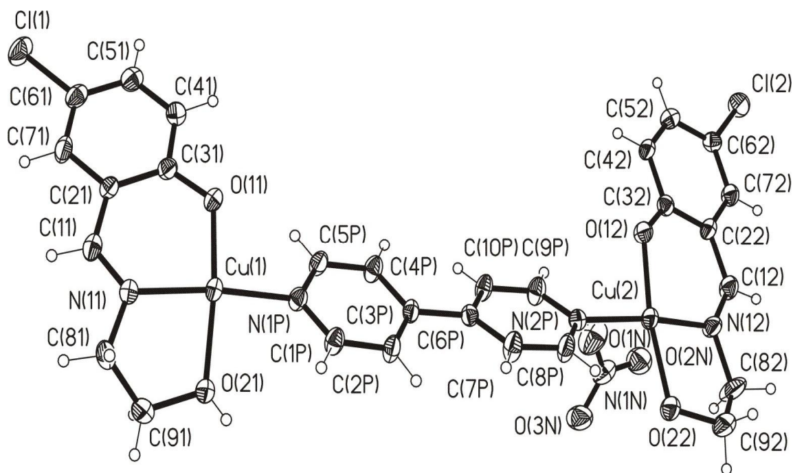
Fig. 1. Structura dimerului în complex și numerotarea atomilor
