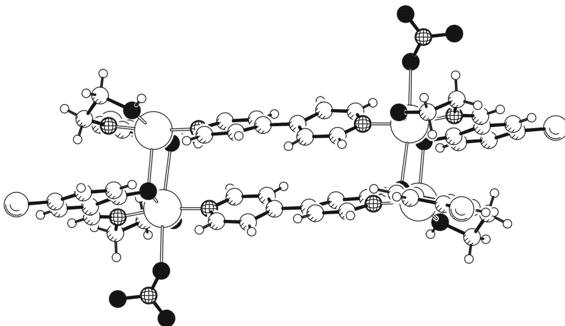
Fig. 2. Formarea tetramerului în complex
