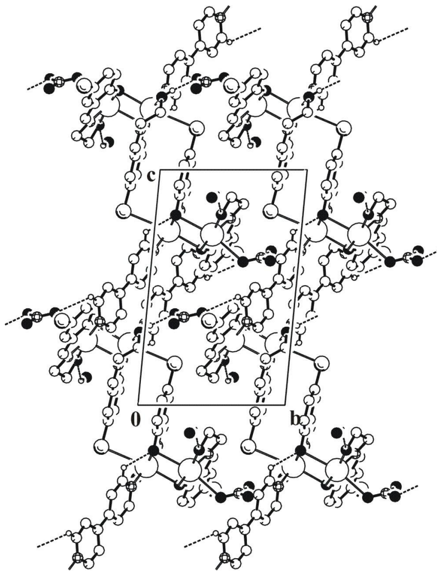
Fig. 3. Un fragment de împachetare al compusului
